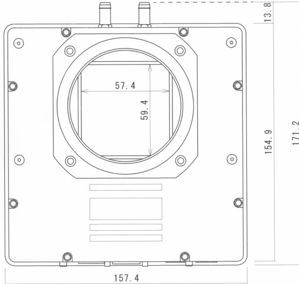
STX • 正面図 (単位：m/m)
